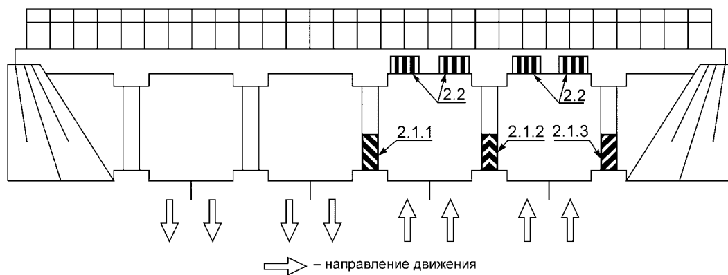
Рисунок В.22 - Пример нанесения разметки 2.1 и 2.2
