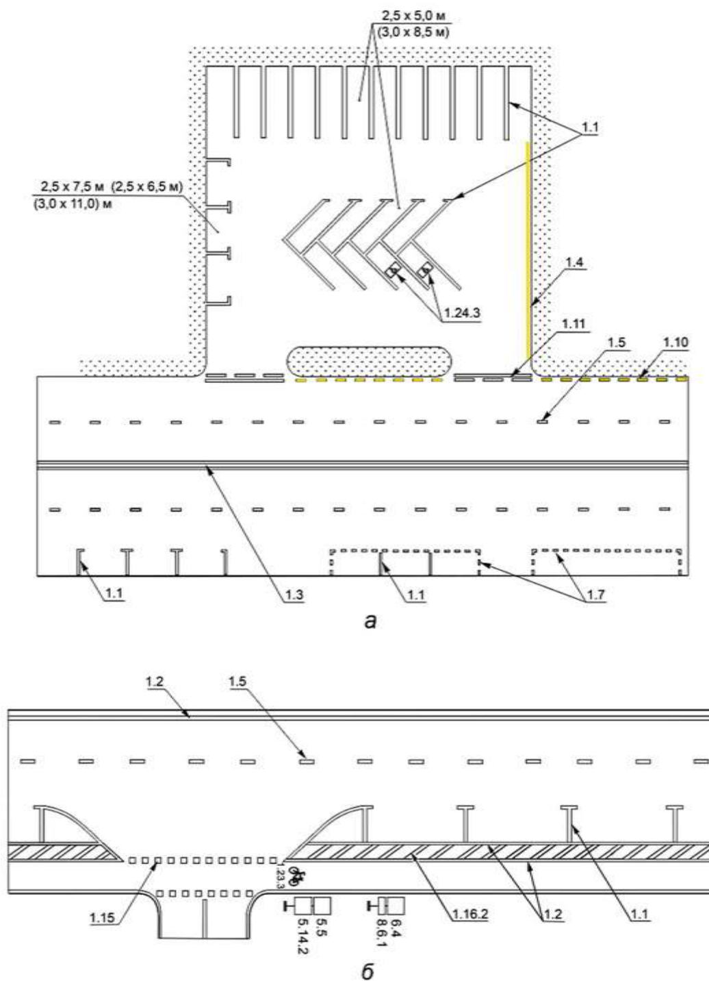
Рисунок В.12 - Пример нанесения разметки 1.16.1 - 1.16.3
