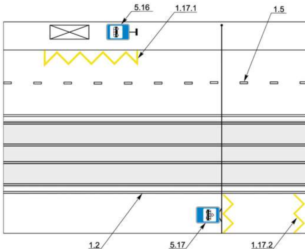
Рисунок В.15 - Пример нанесения разметки 1.17.1 и 1.17.2
