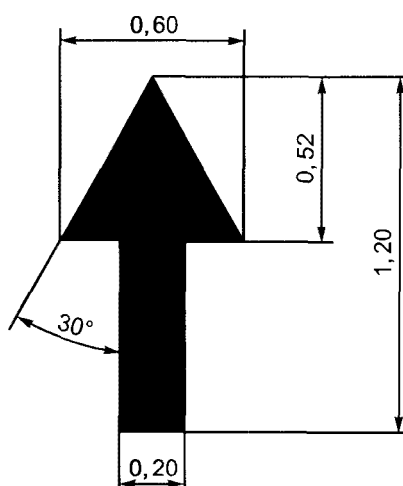
Рисунок Б.3 - Размеры стрел на разметке 1.14.2
