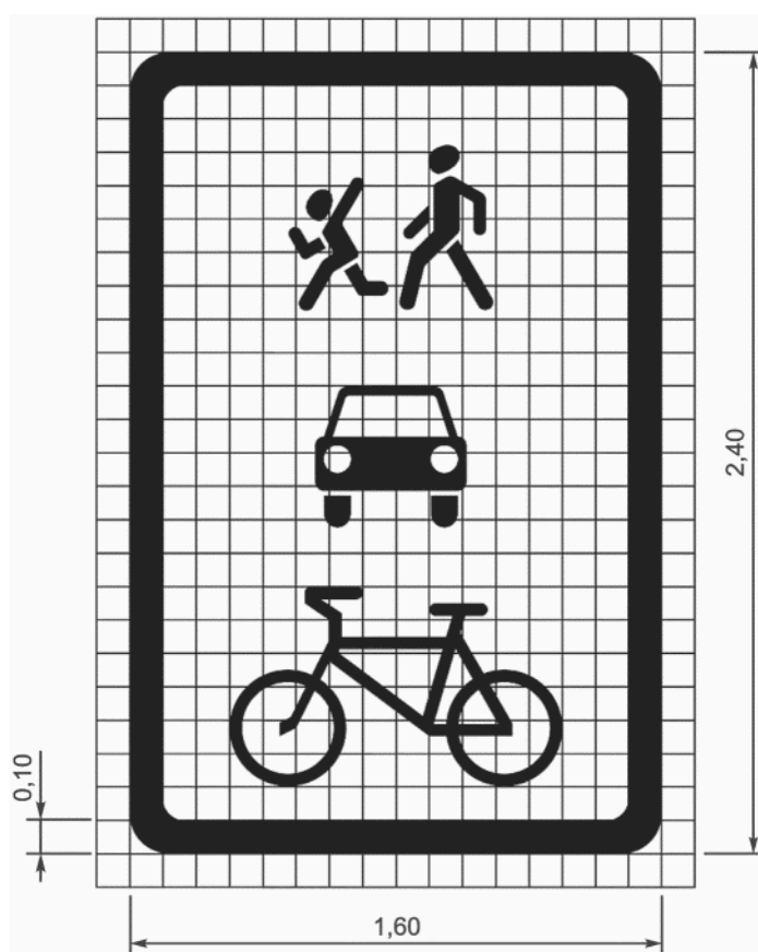
Рисунок Б.19 - Размеры разметки 1.24.6 (рисунок Б.19 введен Изменением N 1 , утв. Приказом Росстандарта от 03.11.2020 N 1024-ст)
