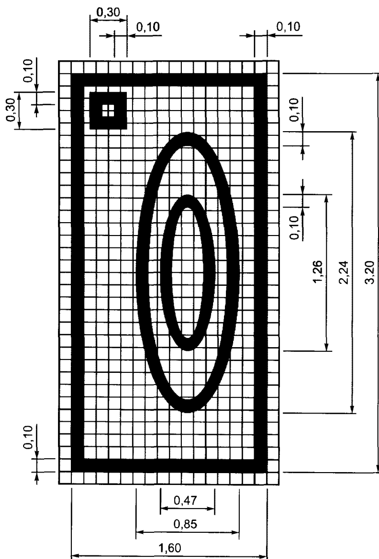
Рисунок Б.17 - Размеры разметки 1.24.4
