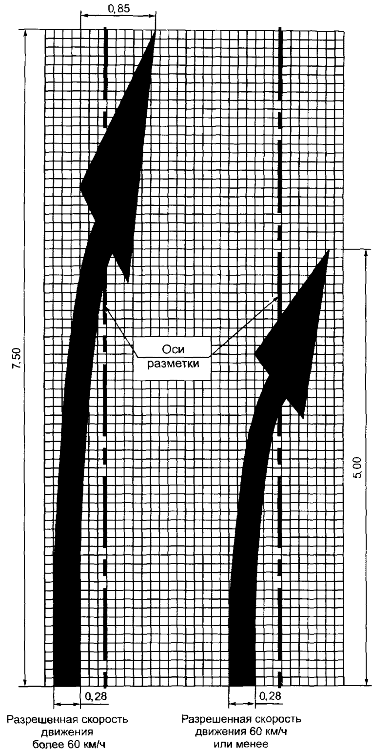
Рисунок Б.6 - Расположение и размеры стрел
