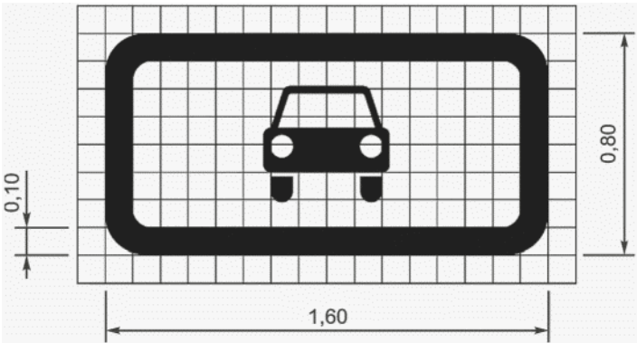
Рисунок Б.20 - Размеры разметки 1.24.7 (рисунок Б.20 введен Изменением N 1 , утв. Приказом Росстандарта от 03.11.2020 N 1024-ст)
